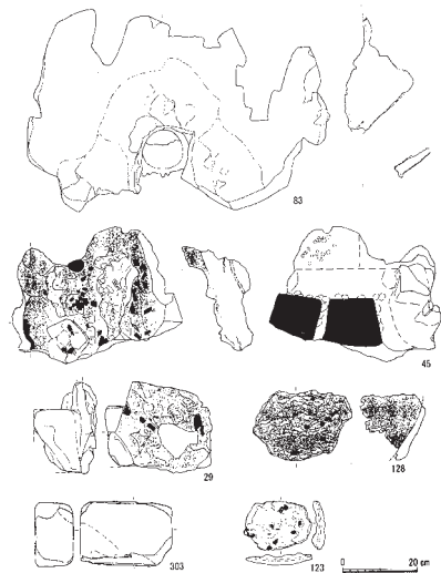
図8 鍛冶屋敷遺跡出土炉壁
