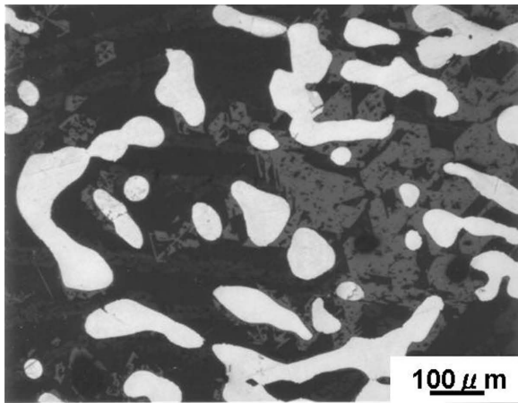
写真6 No. 1位置の小さな粒状鉄のミクロ組織
