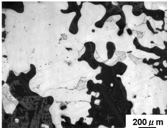
写真7 No. 1位置の粗大な粒状鉄の組織
