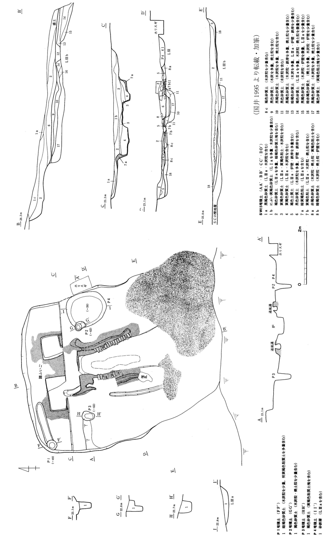
図2 15号製鉄炉 (2)
