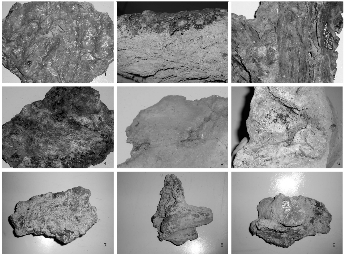
鳥打沢 A 15・16 号 1 炉壁内面 2 炉壁断面 3 発泡洋木炭痕 大迫 5 号 4 炉壁内面 5 炉壁裏側 6 送風孔側面 鳥打沢 A 15・16 号第 12 図 13 7 炉壁内面 8 側面 9 裏側 (1～3、7～9 原町 IX、4～6 原町 VIII)
