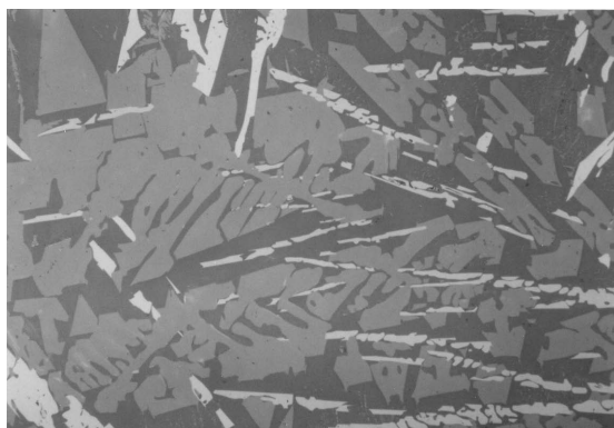
写真 42 顕微鏡写真 (資料 NO. 3-3) × 400
