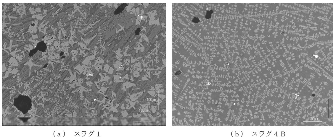
図8 製錬滓試料の光学顕微鏡観察像
