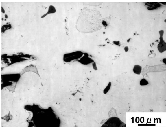
写真8 No. 2位置の粗大な粒状鉄のミクロ組織
